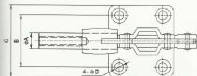
GH-305-HM M12×35
